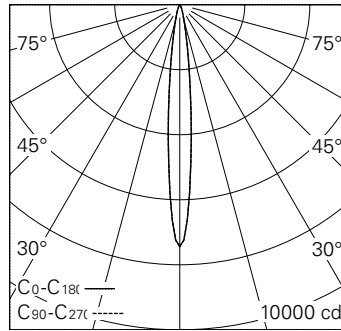
LED 2700 K 9,3 W 531 lm-h 11.0° / CIE Flux 99 100 100 100 / A80 nach DIN 5040
