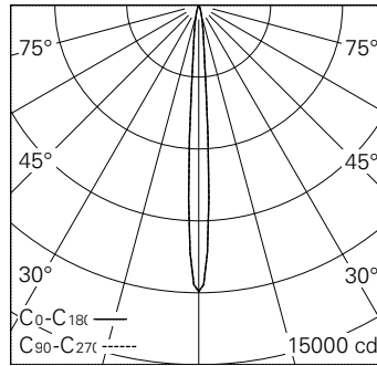
LED 3000 K 9,3 W 475 lm-h 7.6° / CIE Flux 99 100 100 100 100 / A80 nach DIN 5040
