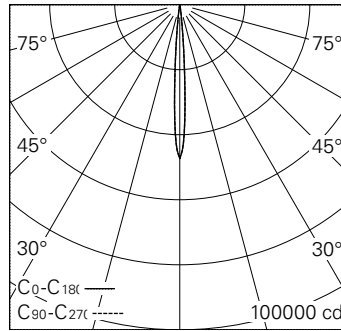
LED 3000 K 20 W 1037 lm-h 7.4° / CIE Flux 99 100 100 100 / A80 nach DIN 5040
