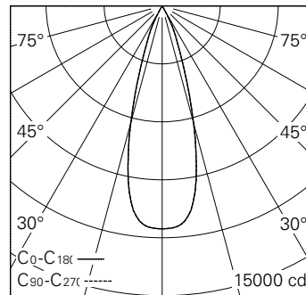
LED 2700 K 42 W 3426 lm-h 32° / CIE Flux 100 100 100 100 100 / A80 nach DIN 5040
