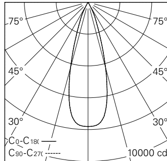
LED 4000 K 20 W 2319 lm-h 32° / CIE Flux 100 100 100 100 100 / A80 nach DIN 5040
