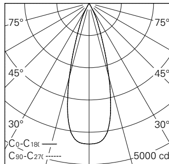
LED 2700 K 14 W 1297 lm-h 32° / CIE Flux 100 100 100 100 100 / A80 nach DIN 5040
