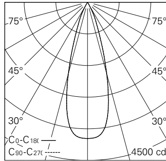
LED 3000 K 14 W 1151 lm-h 32° / CIE Flux 100 100 100 100 100 / A80 nach DIN 5040
