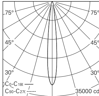
LED 3000 K 27 W 2303 lm-h 12.0° / CIE Flux 100 100 100 100 100 / A80 nach DIN 5...
