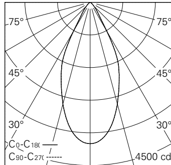
LED 4000 K 20 W 2399 lm-h 48° / CIE Flux 94 99 100 100 100 / A80 nach DIN 5040
