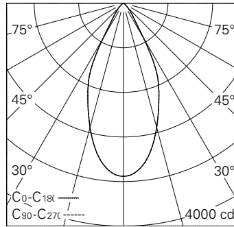
LED 3000 K 20 W 1910 lm-h 48° / CIE Flux 94 99 100 100 100 / A80 nach DIN 5040
