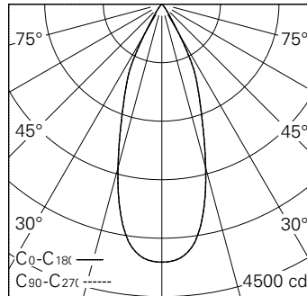
LED 3000 K 20 W 1770 lm-h 38° / CIE Flux 98 100 100 100 100 / A80 nach DIN 5040
