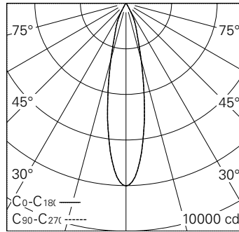
LED 2700 K 20 W 1819 lm-h 22° / CIE Flux 98 100 100 100 100 / A80 nach DIN 5040
