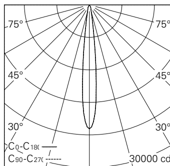
LED 3000 K 20 W 1706 lm-h 12.0° / CIE Flux 100 100 100 100 100 / A80 nach DIN 5...
