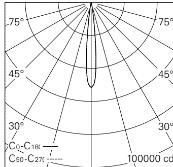
LED 4000 K 31 W 2514 lm-h 11.8° / CIE Flux 99 100 100 100 / A80 nach DIN 5040
