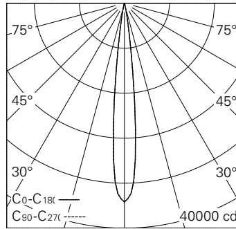
LED 3000 K 31 W 1721 lm-h 11.8° / CIE Flux 99 100 100 100 100 / A80 nach DIN 5040
