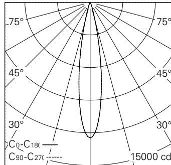
LED 3000 K 20 W 1510 lm-h 18.6° / CIE Flux 99 100 100 100 / A80 nach DIN 5040
