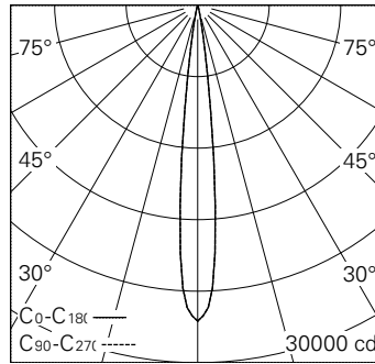
LED 2700 K 20 W 1291 lm-h 11.8° / CIE Flux 99 100 100 100 100 / A80 nach DIN 5040
