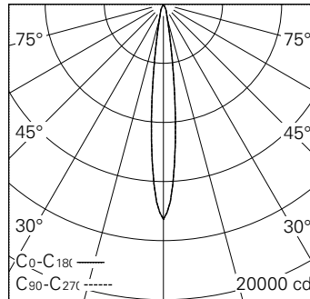
LED 2700 K 13,7 W 1137 lm-h 12.6° / CIE Flux 100 100 100 100 100 / A80 nach DIN...
