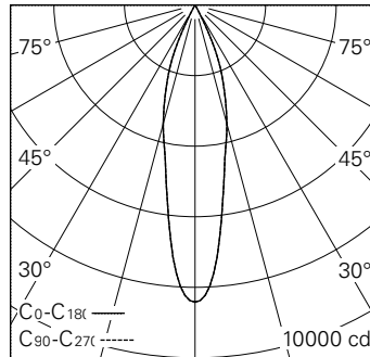
LED 4000 K 20 W 2064 lm-h 24° / CIE Flux 100 100 100 100 100 / A80 nach DIN 5040
