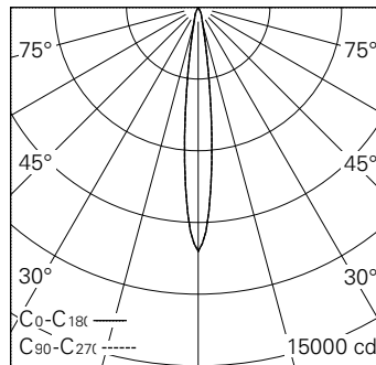
LED 3000 K 11 W 797 lm-h 12.6° / CIE Flux 100 100 100 100 100 / A80 nach DIN 5040
