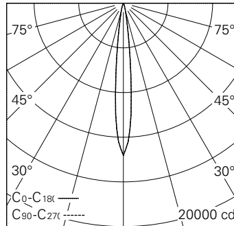
LED 2700 K 11 W 862 lm-h 11.6° / CIE Flux 100 100 100 100 100 / A80 nach DIN 5040
