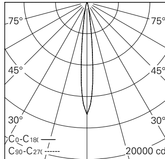
LED 3000 K 11 W 902 lm-h 11.6° / CIE Flux 100 100 100 100 100 / A80 nach DIN 5040
