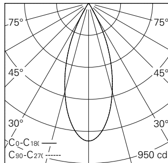
LED 2700 K 11 W 348 lm-h 38° / CIE Flux 99 100 100 100 100 / A80 nach DIN 5040
