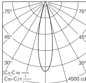
LED 4000 K 11 W 686 lm-h 22° / CIE Flux 99 100 100 100 100 / A80 nach DIN 5040
