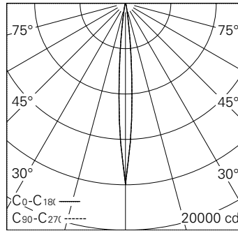
LED 3000 K 11 W 584 lm-h 8.2° / CIE Flux 100 100 100 100 100 / A80 nach DIN 5040
