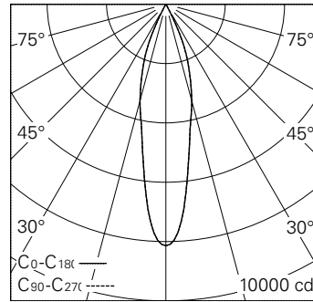
LED 3000 K 19,5 W 1995 lm-h 24° / CIE Flux 100 100 100 100 100 / A80 nach DIN 5...
