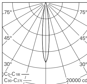
LED 2700 K 13,7 W 1137 lm-h 12.6° / CIE Flux 100 100 100 100 100 / A80 nach DIN...
