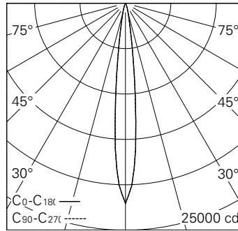
LED 3000 K 19,5 W 1394 lm-h 11.6° / CIE Flux 100 100 100 100 / A80 nach DIN...
