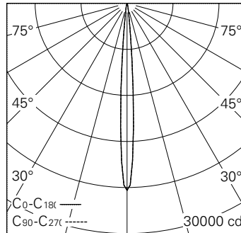
LED 3000 K 11 W 692 lm-h 7.6° / CIE Flux 100 100 100 100 100 / A80 nach DIN 5040
