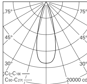
LED 4000 K 42 W 4427 lm-h 32° / CIE Flux 100 100 100 100 100 / A80 nach DIN 5040
