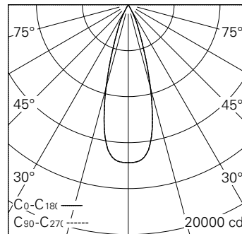
LED 4000 K 36 W 4083 lm-h 32° / CIE Flux 100 100 100 100 100 / A80 nach DIN 5040
