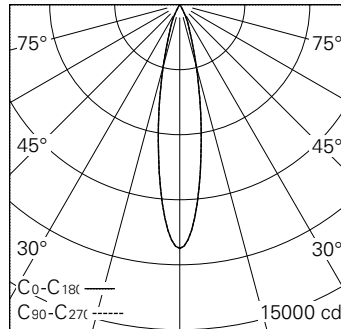
LED 3000 K 27 W 2019 lm-h 20° / CIE Flux 98 100 100 100 100 / A80 nach DIN 5040
