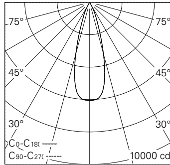
LED 2700 K 20 W 1798 lm-h 32° / CIE Flux 100 100 100 100 100 / A80 nach DIN 5040
