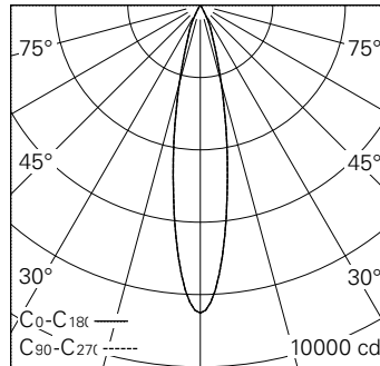
LED 3000 K 20 W 1528 lm-h 20° / CIE Flux 98 100 100 100 100 / A80 nach DIN 5040
