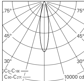
LED 3000 K 14 W 1135 lm-h 20° / CIE Flux 98 100 100 100 100 / A80 nach DIN 5040
