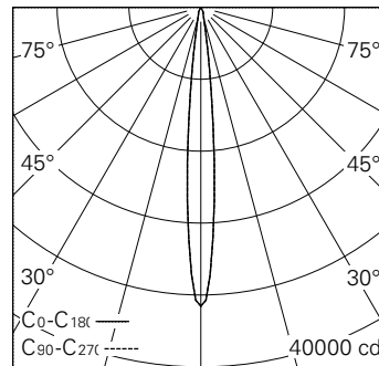
LED 4000 K 14 W 1817 lm-h 10.2° / CIE Flux 100 100 100 100 100 / A80 nach DIN 5...
