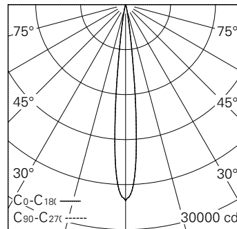
LED 2700 K 20 W 1351 lm-h 11.6° / CIE Flux 96 100 100 100 100 / A80 nach DIN 5040
