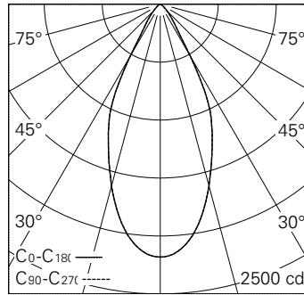
LED 2700 K 14 W 1342 lm-h 48° / CIE Flux 94 99 100 100 100 / A80 nach DIN 5040
