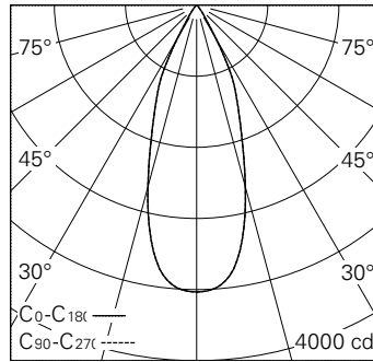
LED 2700 K 14 W 1439 lm-h 38° / CIE Flux 98 100 100 100 100 / A80 nach DIN 5040
