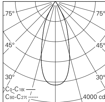
LED 3000 K 14 W 1480 lm-h 38° / CIE Flux 98 100 100 100 100 / A80 nach DIN 5040
