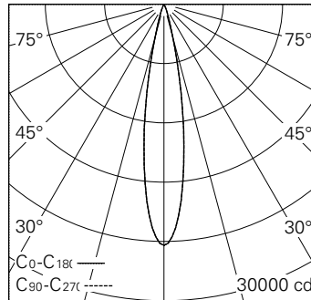
LED 4000 K 27 W 2954 lm-h 18.6° / CIE Flux 99 100 100 100 / A80 nach DIN 5040
