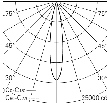
LED 3000 K 27 W 2334 lm-h 18.6° / CIE Flux 99 100 100 100 100 / A80 nach DIN 5040
