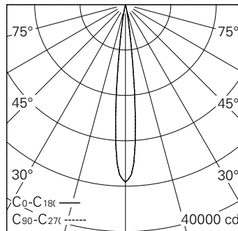
LED 3000 K 27 W 1523 lm-h 11.8° / CIE Flux 99 100 100 100 / A80 nach DIN 5040
