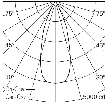
LED 2700 K 20 W 1720 lm-h 38° / CIE Flux 99 100 100 100 100 / A80 nach DIN 5040
