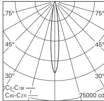
LED 3000 K 20 W 1411 lm-h 12.6° / CIE Flux 100 100 100 100 100 / A80 nach DIN 5...
