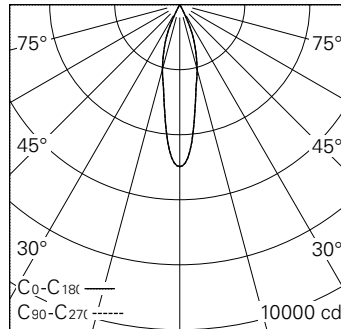
LED 3000 K 14 W 1221 lm-h 24° / CIE Flux 100 100 100 100 100 / A80 nach DIN 5040
