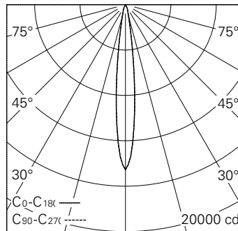
LED 2700 K 14 W 1137 lm-h 12.6° / CIE Flux 100 100 100 100 100 / A80 nach DIN 5...
