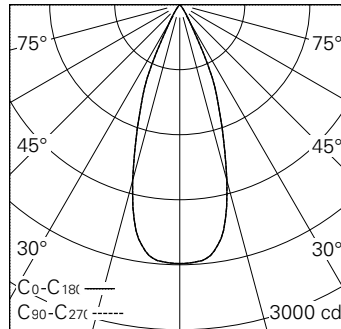
LED 3000 K 11 W 1012 lm-h 38° / CIE Flux 99 100 100 100 100 / A80 nach DIN 5040
