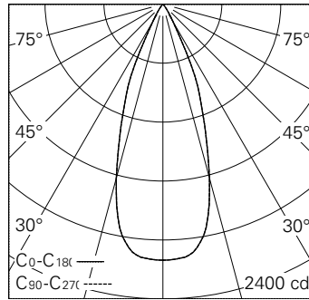
LED 3000 K 11 W 883 lm-h 38° / CIE Flux 99 100 100 100 100 / A80 nach DIN 5040
