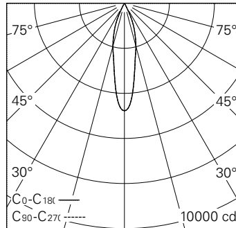
LED 4000 K 11 W 1170 lm-h 24° / CIE Flux 100 100 100 100 100 / A80 nach DIN 5040
